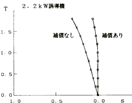
図3 すべり補償特性
